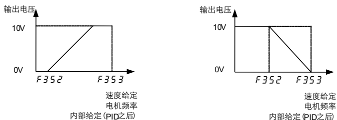
图 6.19 F352 和 F353 设置示意图
