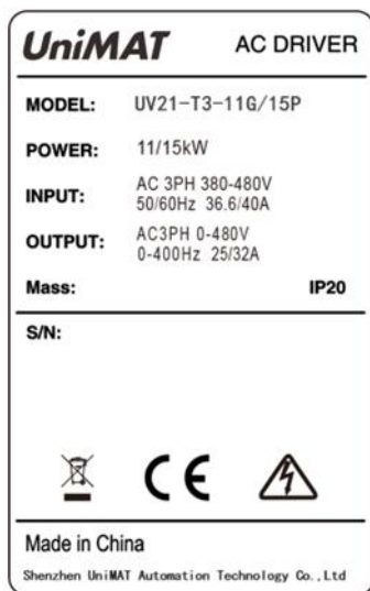
图 3.2 铭牌示例
