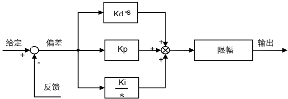
图 6.37 PID 调节器框图
