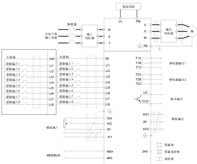
(c) T3 其他标准接线图
