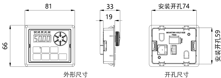
(c) 操作面板带托盘安装尺寸图
