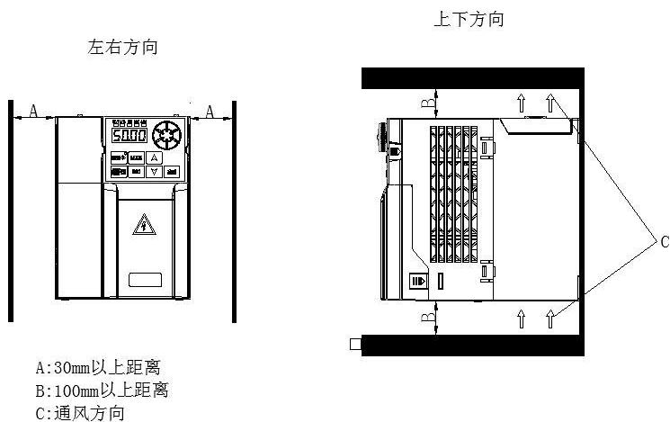
图 4.2 单台安装间距要求
