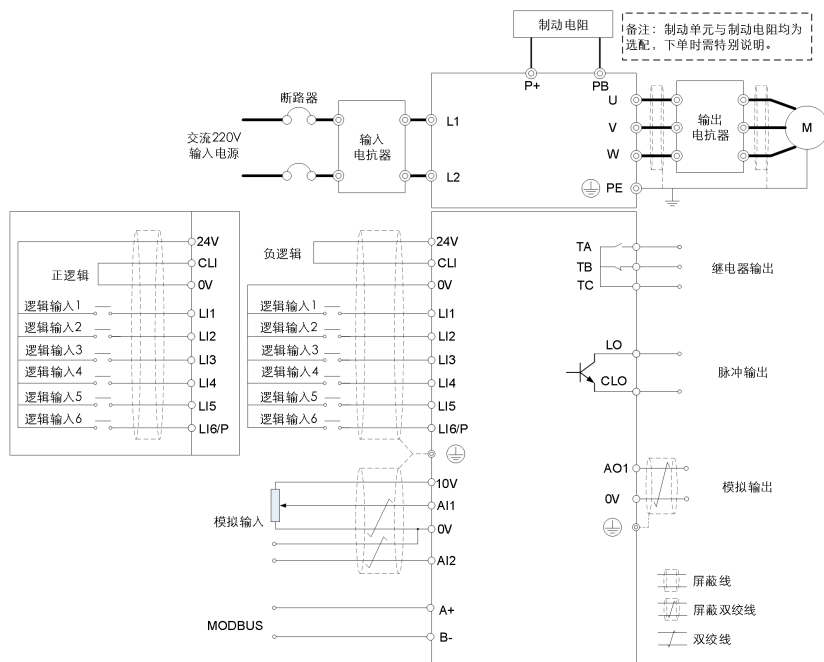
(a) S2 全部标准接线图
