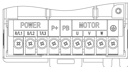
(b) T3-(0R4G -1R5G)主回路功率端子
