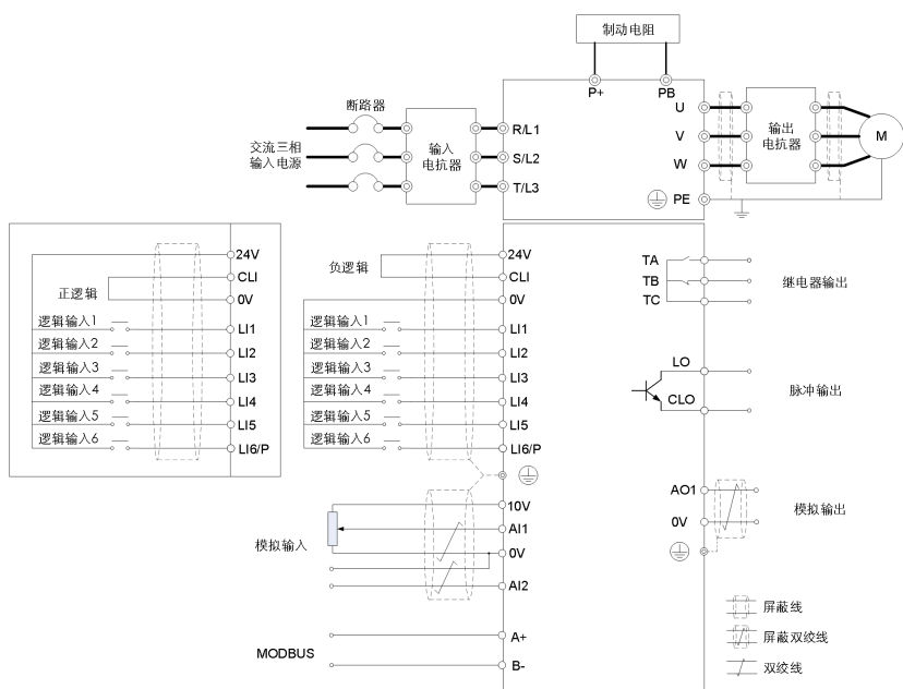
(b) T3-(0R4G-1R5G)标准接线图
