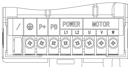
(a) S2 全部主回路功率端子
