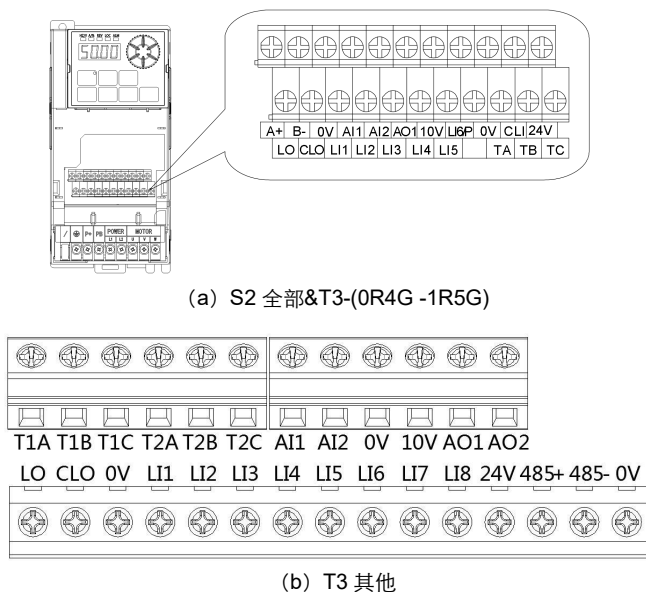
图 4.7 控制端子结构示意图表
