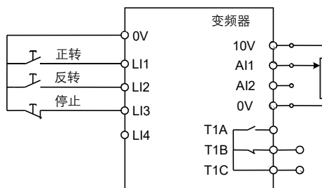
图 5.8 3 线控制 (负逻辑) 接线示意图
