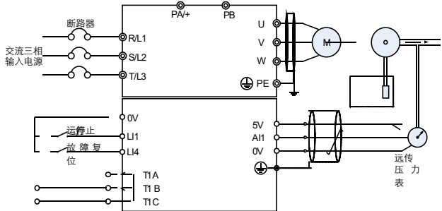
图 6.38 PID 外部连接示例
