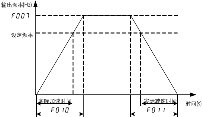
图 6.3 加速时间和减速时间定义
