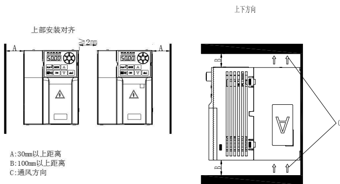
图 4.3 多台左右安装间距要求
