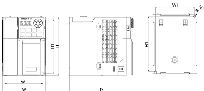
(b) T3 其他
