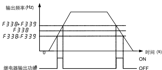
图 6.14 继电器输出-频率检出 2 示意图
