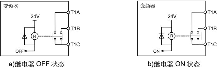
图 6.10 继电器状态说明
