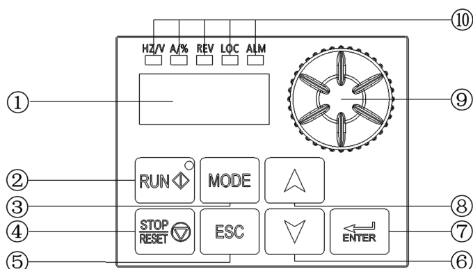
图 5.1 操作面板外形
