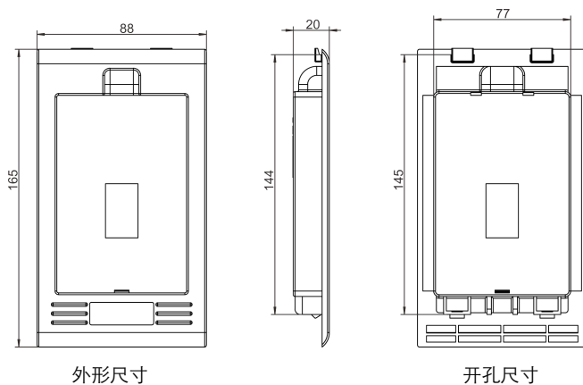
图 3.3 操作面板尺寸图
