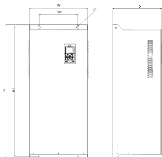
图 3.5 外形及安装尺寸图 (三相含 铁壳 15kW-315kW)
