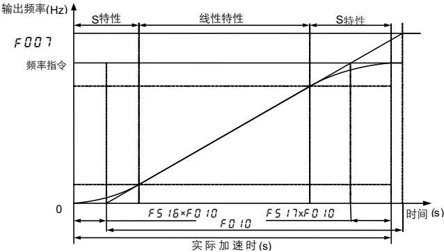
图 6.28 S 型曲线 1
