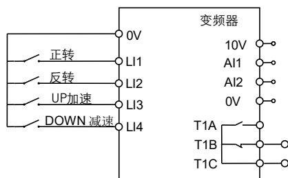
图 5.9 UP/DOWN 加减速接线示意图
