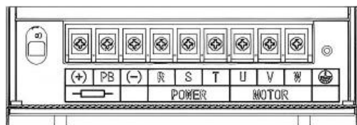
(f) 主回路功率端子 (30-37kW)
