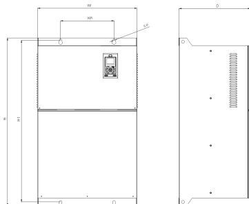
图 3.6 外形及安装尺寸图 (三相含 355kW-500kW)
