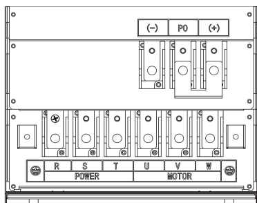
(i) 主回路功率端子 (75-110kW)
