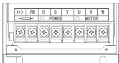
(d) 主回路端子(铁壳15-18kW)
