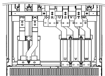
(n) 主回路功率端子 (560-800kW)
