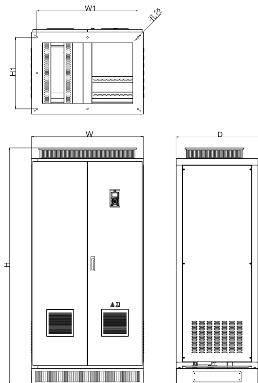
图 3.7 外形及安装尺寸示意图（三相 560kW（含）以上）
