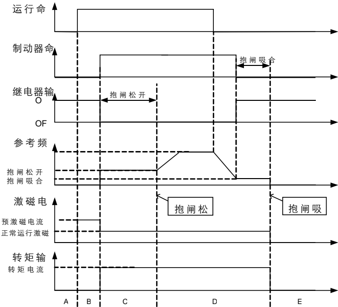
图 6.35 制动器逻辑时序示意图
