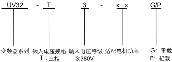
图 3.1 变频器型号说明示意图
