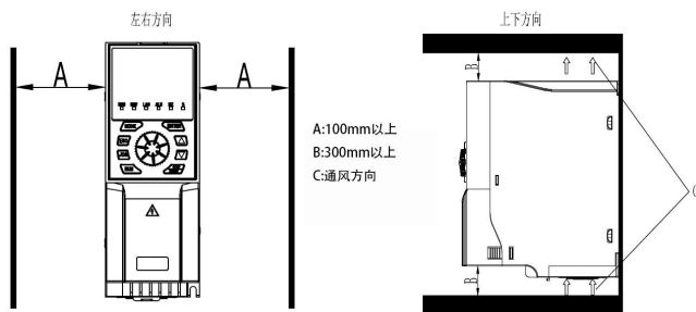
图 4.2 单台安装间距要求
