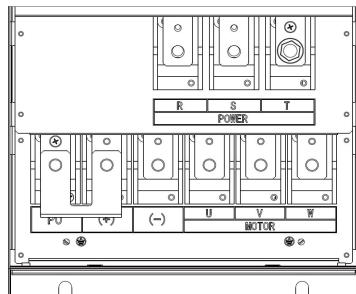
(j) 主回路功率端子 (132-185kW)
