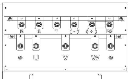
(m) 主回路功率端子 (355-500kW)
