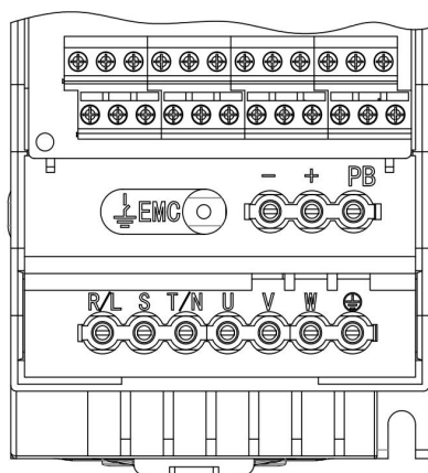
(a) 主回路功率端子 (0.75-3kW)
