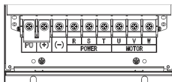
(h) 主回路功率端子 (55kW)
