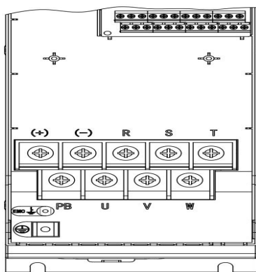
(c) 主回路功率端子 (11-15kW 塑壳)
