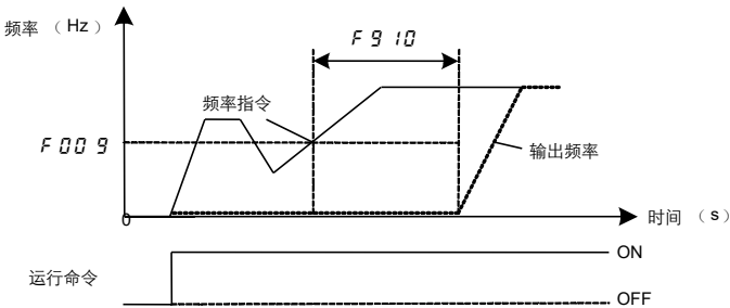
图 6.39 休眠唤醒示意图
