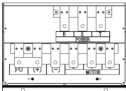
(k) 主回路功率端子 (200-220kW)
