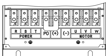
(g) 主回路功率端子 (45kW)
