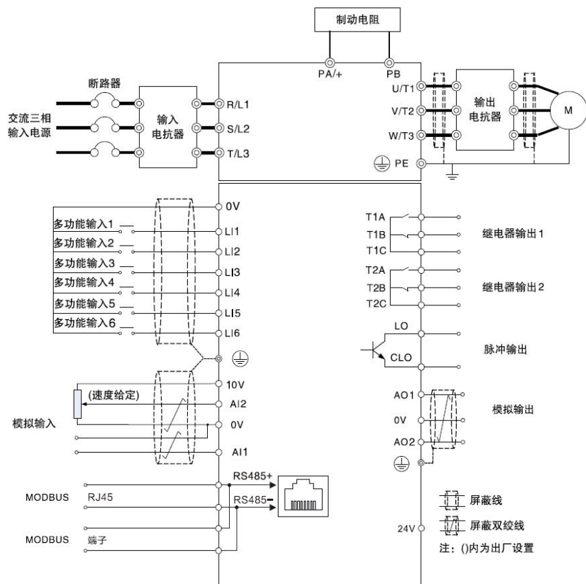
(a) 塑壳 15kW (含) 以下标准接线图
