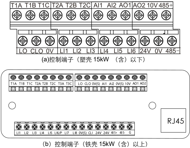
图 4.8 控制端子结构示图
