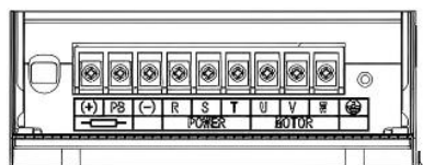
(e) 主回路功率端子 (22kW)
