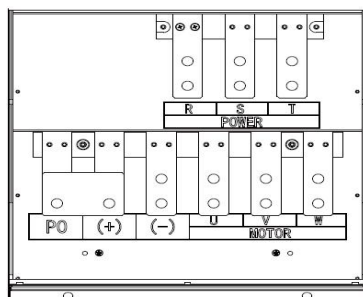
(l) 主回路功率端子 (250-315kW)
