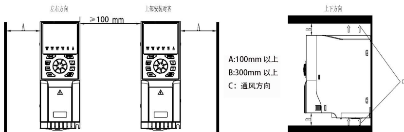
图 4.3 多台左右安装间距要求
