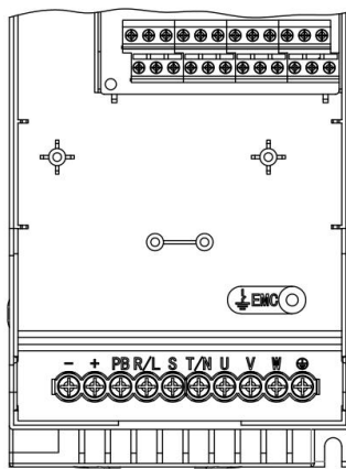
(b) 主回路功率端子 (4-7.5kW)
