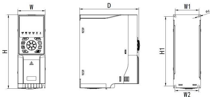
图 3.4 外形及安装尺寸图（三相塑壳 15kW（含）以下）
