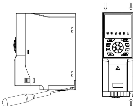
图 4.5 盖板、出线板的拆卸示意图
