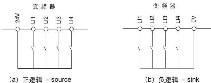
图 4.10 逻辑输入端子接线图
