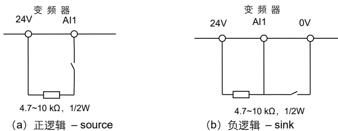
图 4.9 AI1 配置为逻辑输入端子时的接线图
